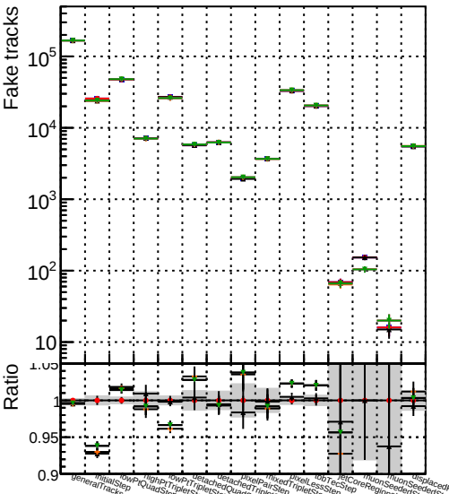
DGM original originalvector_1000evt DGM original 1000evt DGM fitted4_1000evt DGM fit cpeak_1000evt DGM fit cpeak SORTBZ2_1000evt DGM fit cpeak SORTBZ2 TESTOUTLIER5_1000evt
