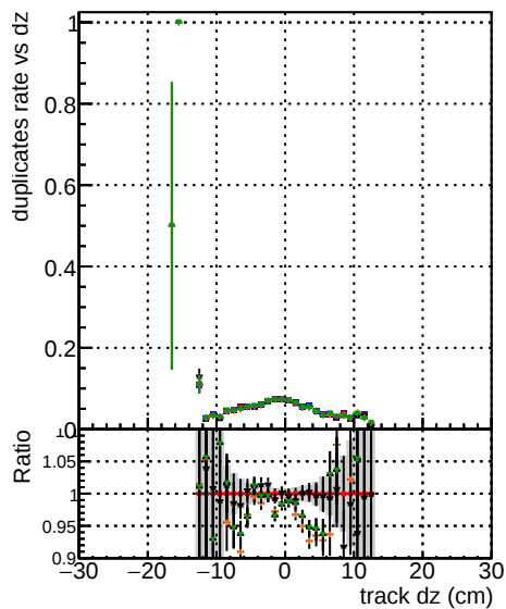
SIGOUTLIER5 1000evt
