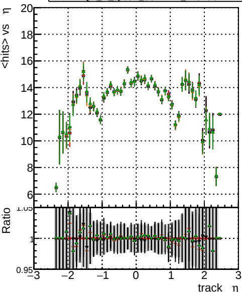
mean hits vs \eta Legend: BGM original original vector 1000evt, BGM fitted 1000evt, BGM fit cpeok SORTRZZ 1000evt, BGM fit cpeok SORTRZZ TESTOUTLIER5 1000evt
