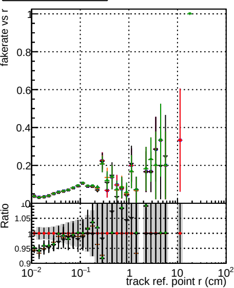
Fake rate vs vertpos DOM original originalvector 1000evt internal 10000evt DOM fit EDCOR SORTRZZ TESTOUTLIER5 1000evt
