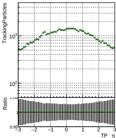
N of sim Legend: DGM original vector_1000evt DGM fitted_1000evt DGM cpeok_1000evt DGM SORTBZ2_1000evt DGM SORTBZ2_TESTOUTLIER5_1000evt
