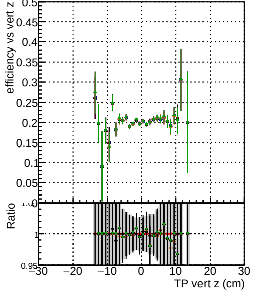
Efficiency vs vert z Legend: - BQM original original vector 1000evt - BQM fitted 1000evt - BQM fit cpeok 1000evt - BQM fit cpeok SORTRZZ 1000evt - BQM fit cpeok SORTRZZ TESTOUTLIER5 1000evt
