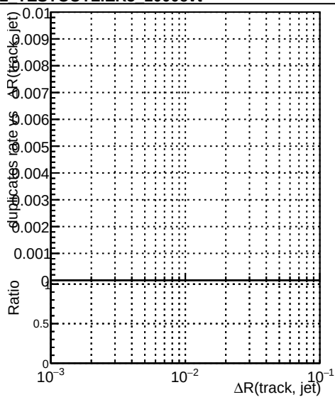
TESTOUTLIER5 1000evt
