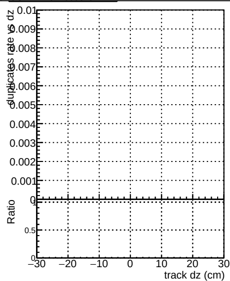
OUTLIER5 1000evt
