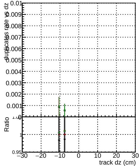
OUTLIER5 1000evt
