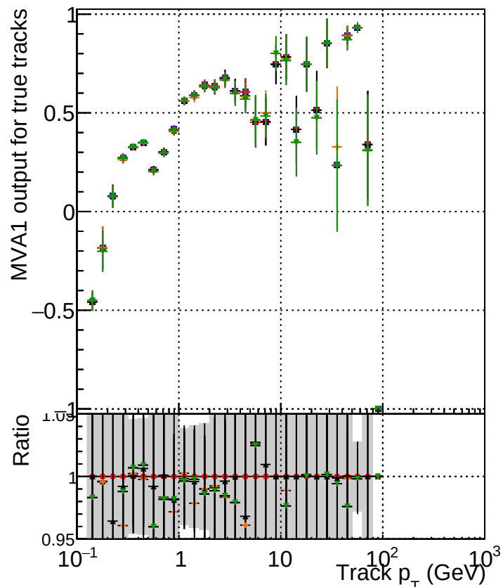
DOM original originalvector_1000evt DOM original_1000evt DOM fitted4_1000evt DOM fit cpeok_1000evt DOM fit cpeok SORTRZ2_1000evt DOM fit cpeok SORTRZ2 TESTOUTLIER5_1000evt
