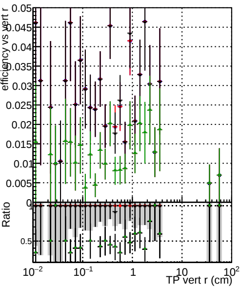
Efficiency vs vertpos Legend: BGM original original vector 1000evt BGM fitted 4 1000evt BGM fitted cpeok SORTZZ 1000evt BGM fitted cpeok SORTZZ TESTOUTLIER5 1000evt
