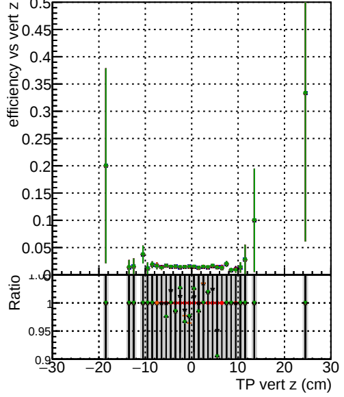
Efficiency vs vert z Legend: - BGM original original vector 1000evt - BGM fitted 4 1000evt - BGM fitted 2 1000evt - BGM fitted cpeok SORTRZZ 1000evt - BGM fitted cpeok SORTRZZ TESTOUTLIER5 1000evt
