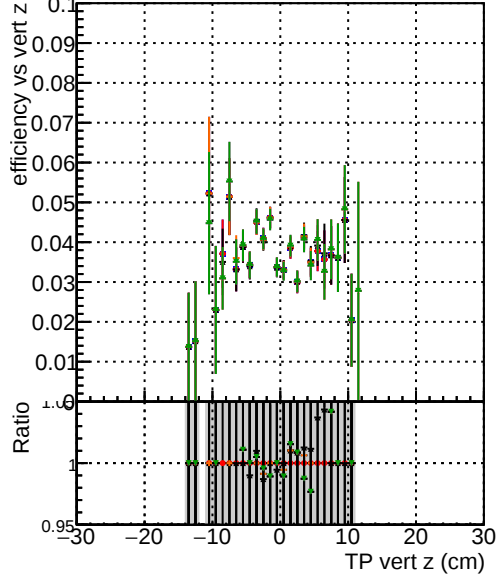
Efficiency vs vert z Legend: - BGM original original vector 1000evt - BGM fitted 4 1000evt - BGM fitted 2 1000evt - BGM fitted 1 1000evt - BGM fitted 0 1000evt - BGM fitted 0 SORTRZZ 1000evt - BGM fitted 0 SORTRZZ TESTOUTLIER5 1000evt
