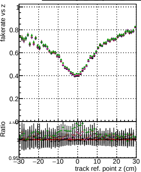
Fake rate vs DOM original 1000evt DOM original 10000evt DOM IL CDF 10000evt DOM IL CDF SORTRZZ 10000evt TESTOUTLIER4 10000evt
