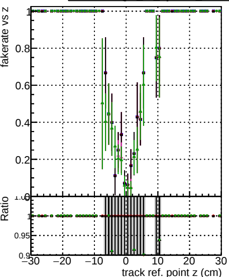
Fake rate vs track ref. point z (cm) DOM original originalvector 1000evt 10000evt 100000evt 1000000evt DOM ILD EDEK SORTRZ2 TESTOUTLIER4 1000evt
