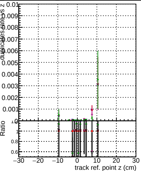
Fake rate vs vertpos Duplicates Rate vs vertpos Pileup rate vs vertpos DOM original originalvector 1000evt 10000evt 100000evt 1000000evt 10000000evt TESTOUTLIER4 1000evt
