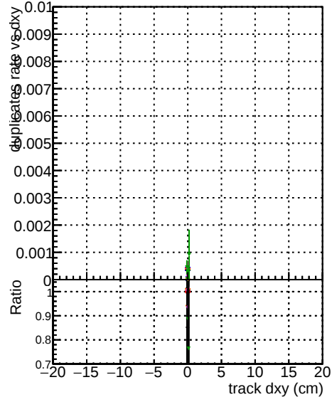
SPROUTLIER4 1000evt
