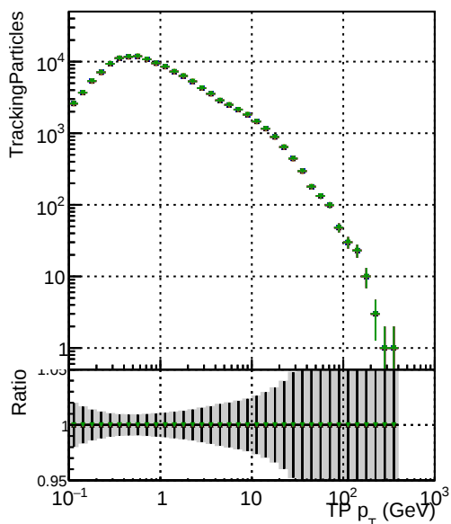
DCM original originalvector_1000evt DCM original 1000evt DCM fitted 1000evt DCM fit cpeak 500evt DCM fit cpeak SORTRZ2 1000evt DCM fit cpeak SORTRZ2 TESTOUTLIER4 1000evt
