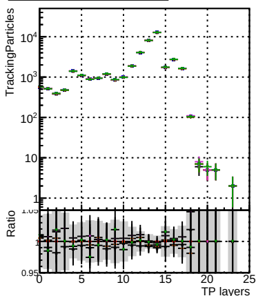
N of sim Legend DQM_fit_cpeOK_1000evl DQM_fit_cpeOK_SORTRZ DQM_fit_cpeOK_SORTRZ
