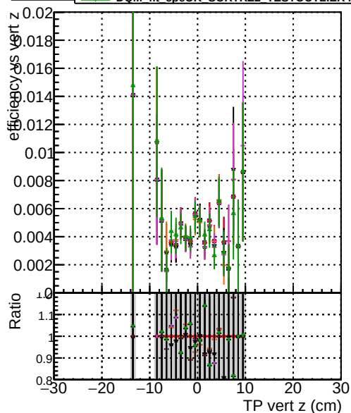
Efficiency Legend: DOM original 1000evt DOM original vector 1000evt DOM fitted 4 1000evt DOM fit cpeok 1000evt DOM fit cpeok SORTBZ2 1000evt DOM fit cpeok SORTBZ2 TESTOUTLIER4 1000evt
