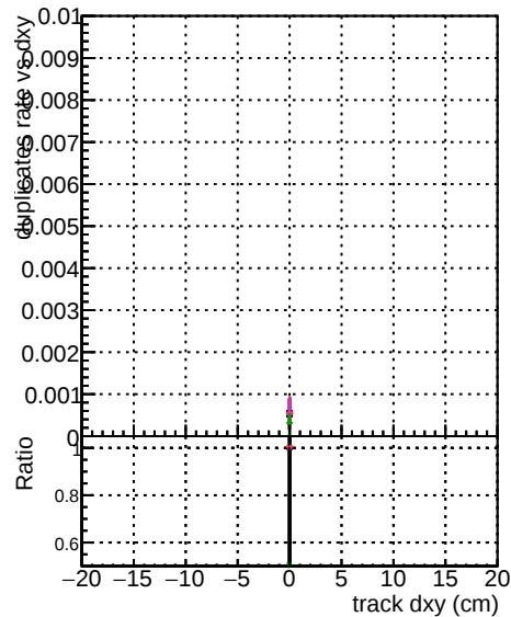
OUTLIER4 1000evt
