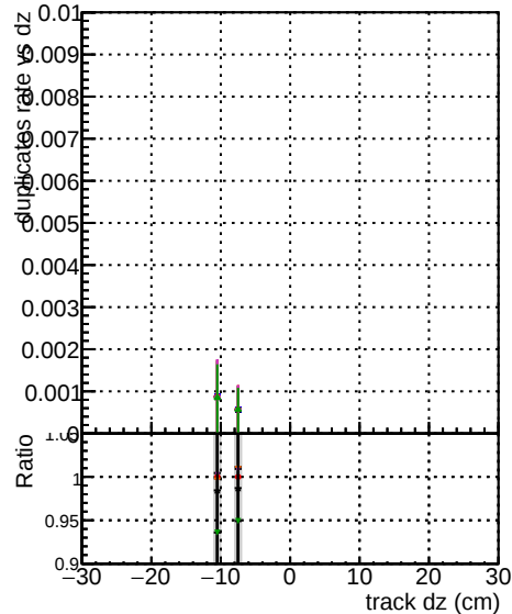
OUTLIER4 1000evt
