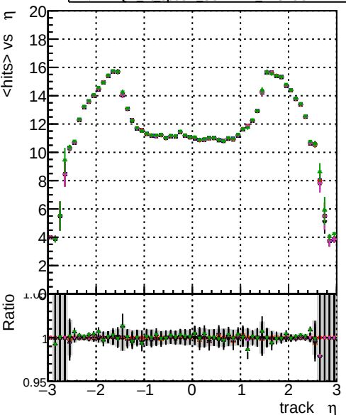
mean hits vs \eta Legend: - BGM original vector 1000evt - BGM fitted 4 1000evt - BGM fit cpeok SORTRZZ 1000evt - BGM fit cpeok SORTRZZ TESTOUTLIER4 1000evt
