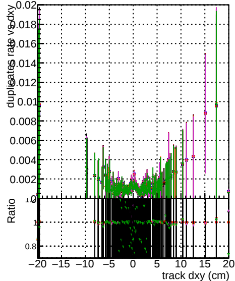
ROUTLIER4 1000evt
