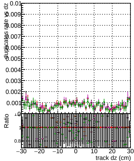
ROUTLIER4 1000evt
