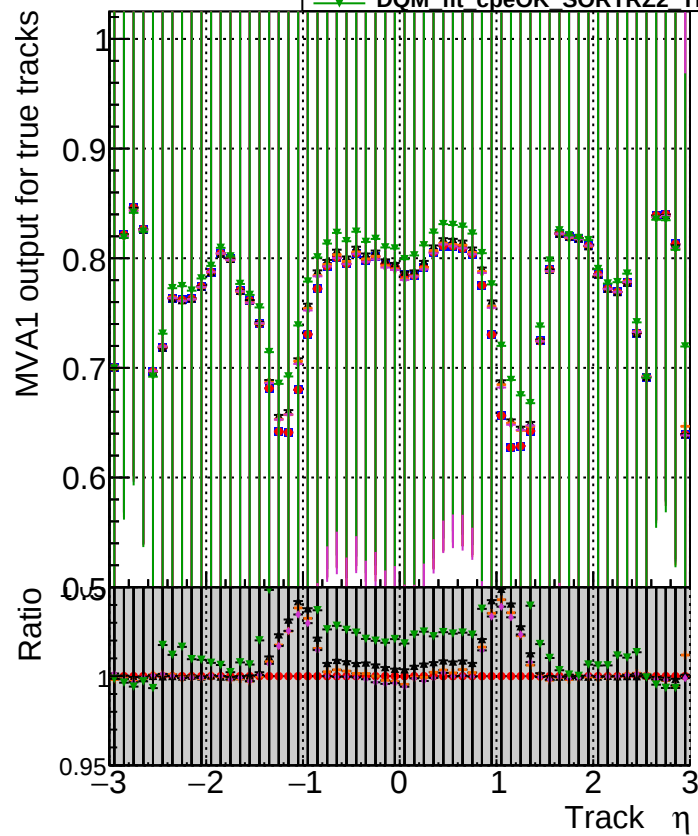
DOM original originalvector_1000evt DOM original_1000evt DOM fitted4_1000evt DOM fit cpeok_1000evt DOM fit cpeok SORTRZ2_1000evt DOM fit cpeok SORTRZ2 TESTOUTLIER4_1000evt
