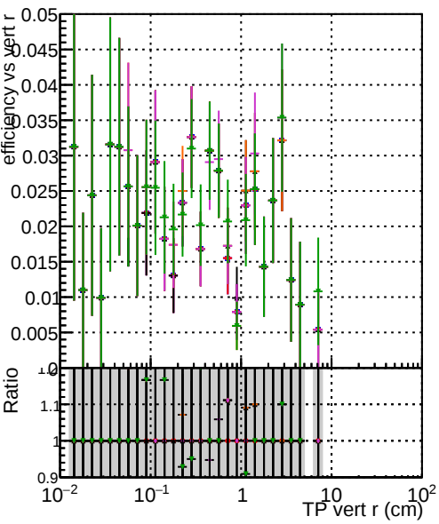
Efficiency vs vertpos Legend: BGM-original BGM-fitted4 BGM-fitted4+1000evt BGM-fitted4+500evt BGM-fitted4+1000evt+500evt BGM-fitted4+1000evt+500evt+1000evt
