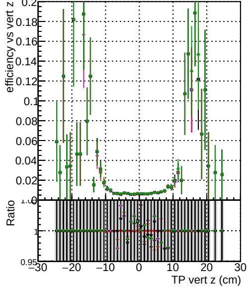
Efficiency vs vert z Legend: BGM original original vector 1000evt, BGM fitted4 1000evt, BGM fittedcpeok 1000evt, BGM fittedSORTRZZ 1000evt, BGM fittedcpeok SORTRZZ TESTOUTLIER4 1000evt
