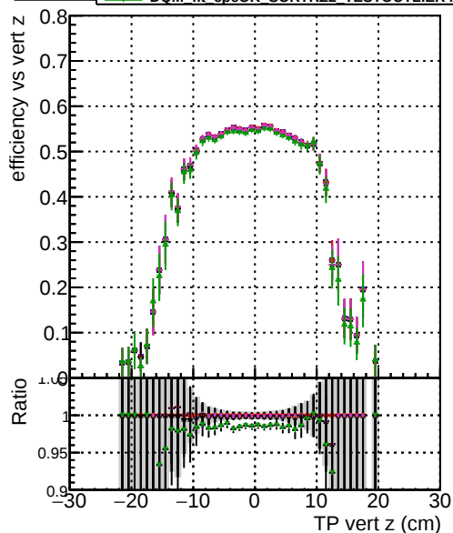
Efficiency Legend: DCM original originalvector_1000evt DCM original 10000evt DCM fitted 10000evt DCM fit cpeok 5000evt DCM fit cpeok SORTRZ2 10000evt DCM fit cpeok SORTRZ2 TESTOUTLIER4 10000evt
