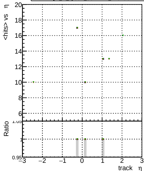
mean hits vs \eta Legend: BGM original vector 1000evt, BGM fitted 4 1000evt, BGM fit cpeok SORTRZZ 1000evt, BGM fit cpeok SORTRZZ TESTOUTLIER4 1000evt
