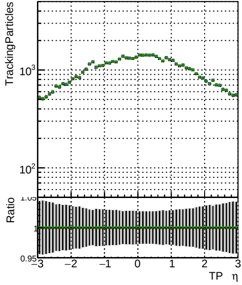
Legend: BGM original original vector 1000evt, BGM fitted4 1000evt, BGM fitted500 500evt, BGM fitted500 SORTRZZ 1000evt, BGM fitted500 SORTRZZ TESTOUTLIER4 1000evt
