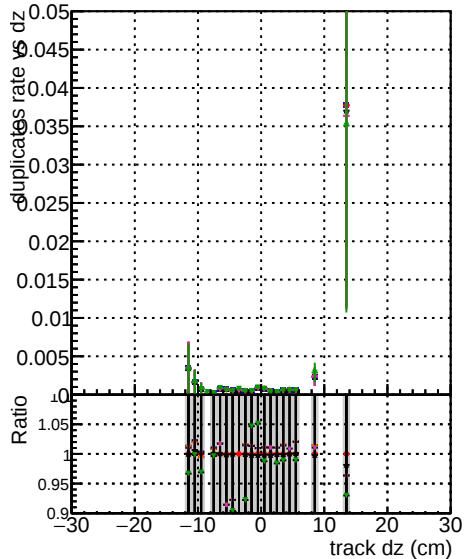
OUTLIER4 1000evt
