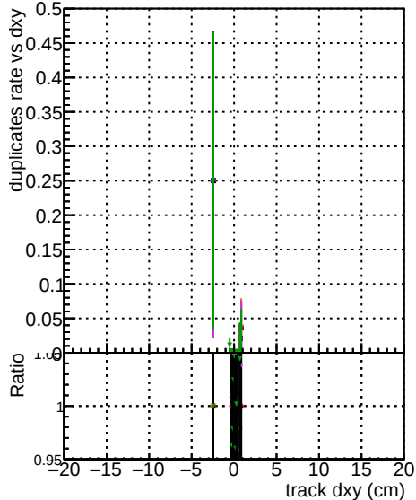
OUTLIER4 1000evt
