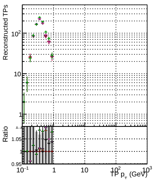
Legend: BGM original original vector 1000evt, BGM fitted 4 1000evt, BGM fitted 2 1000evt, BGM fitted cpeok SORTRZZ 1000evt, BGM fitted cpeok SORTRZZ TESTOUTLIER3 1000evt
