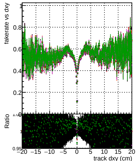
Fake rate vs d DOM original 1000evt DOM original 5000evt DOM original 10000evt DOM in EPOCH SORTR22 1000evt DOM in EPOCH SORTR22 5000evt DOM in EPOCH SORTR22 10000evt
