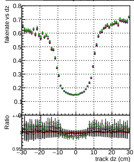
Fake rate vs d DOM original 1000evt DOM original 5000evt DOM original 10000evt DOM in EPOCH SORTR22 1000evt DOM in EPOCH SORTR22 5000evt DOM in EPOCH SORTR22 10000evt
