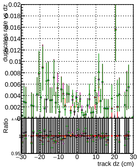
OUTLIER3 1000evt
