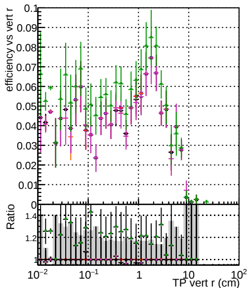
Efficiency Legend: DOM original 1000evt DOM original vector 1000evt DOM fitted 4 1000evt DOM fit cpeok 1000evt DOM fit cpeok SORTBZ2 1000evt DOM fit cpeok SORTBZ2 TESTOUTLIER3 1000evt
