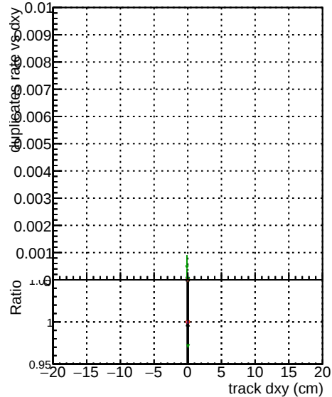
SPROUTLIER3 1000evt
