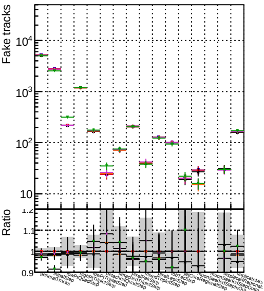
Number Color Model Dataset Configuration 1 Orange DOM fit cpeok-1000evt 2 Orange DOM fit cpeok-SORTRZZ-1000evt 3 Purple DOM fit cpeok-SORTRZZ-TESTOUTLIER3-1000evt 4 Green DOM fit cpeok-SORTRZZ-TESTOUTLIER3-1000evt
