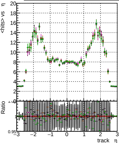
mean hits vs \eta Legend: - BGM original original vector 1000evt - BGM fitted 4 1000evt - BGM fit cpeok SORTZZ 1000evt - BGM fit cpeok SORTZZ TESTOUTLIER3 1000evt
