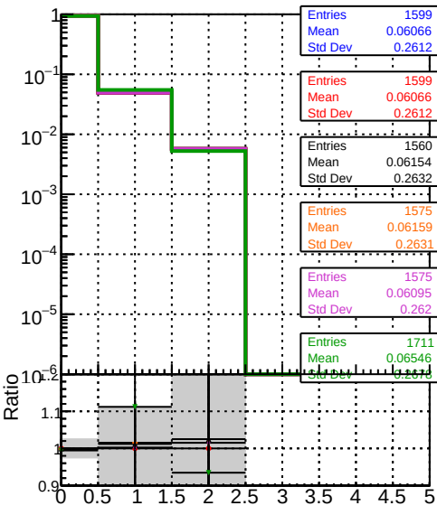
mean hits vs \eta Legend: - BGM original original vector 1000evt - BGM fitted 1000evt - BGM fit cpeok SORTRZZ 1000evt - BGM fit cpeok SORTRZZ TESTOUTLIER3 1000evt
