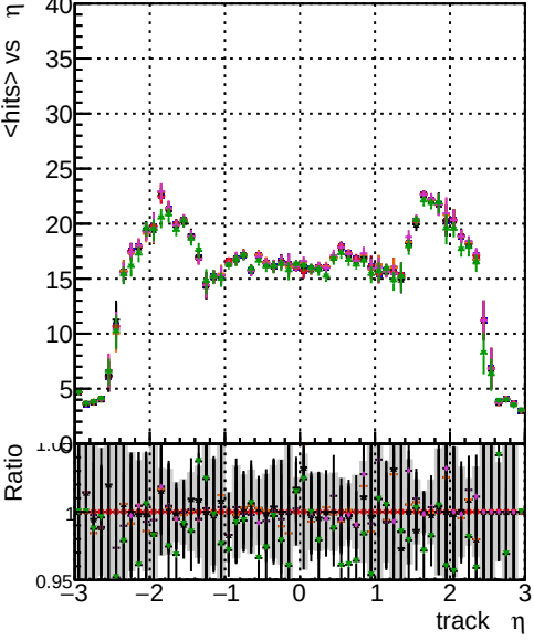
mean hits vs \eta Legend: - BGM original original vector 1000evt - BGM fitted 1000evt - BGM fit cpeok SORTRZZ 1000evt - BGM fit cpeok SORTRZZ TESTOUTLIER3 1000evt
