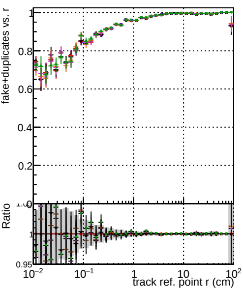
— BQM original original vector 1000evt — BQM fitted 4 1000evt — BQM fitted 2 1000evt — BQM fitted 1 1000evt — BQM fit cpeok SORTRZZ TESTOUTLIER3 1000evt
