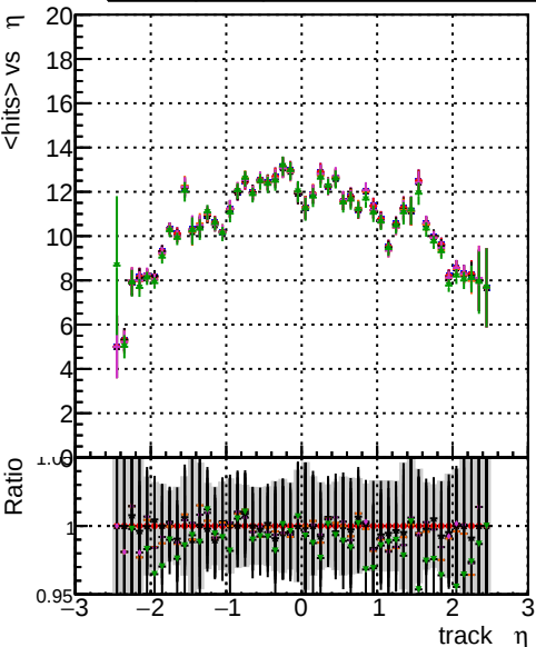
mean hits vs \eta Legend: BGM original vector 1000evt, BGM fitted 1000evt, BGM fit cpeok SORTRZZ 1000evt, BGM fit cpeok SORTRZZ TESTOUTLIER3 1000evt
