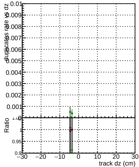
OUTLIER3 1000evt
