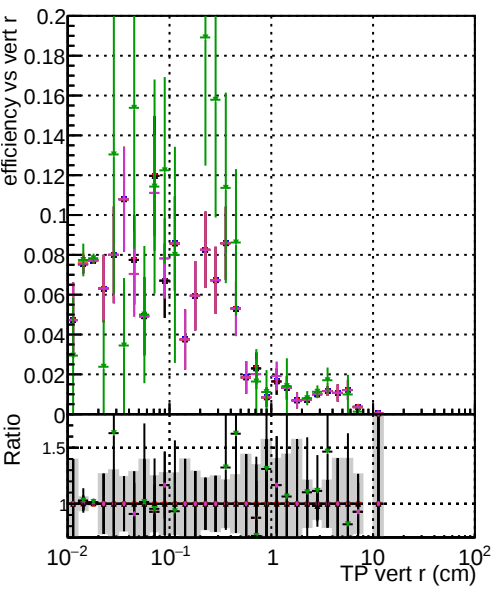
Efficiency vs TP vert r (cm) Legend: original fit original vector 1000evt fit 4 1000evt fit cpeok 1000evt fit cpeok SORTRZZ 1000evt fit cpeok SORTRZZ TESTOUTLIER2 1000evt
