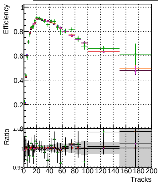
DOM original originalvector_1000evt DOM original_1000evt DOM fitted4_1000evt DOM fit cpeak_1000evt DOM fit cpeak SORTRZ2 1000evt DOM fit cpeak SORTRZ2 TESTOUTLIER2 1000evt
