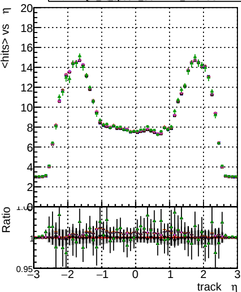
mean hits vs \eta Legend: BGM original original vector 1000evt, BGM fitted 1000evt, BGM fit cpeok SORTRZZ 1000evt, BGM fit cpeok SORTRZZ TESTOUTLIER2 1000evt
