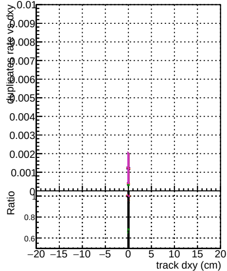
SPROUTLIER2 1000evt
