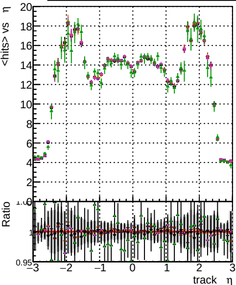
mean hit \eta Legend: - BGM original original vector 1000evt - BGM fitted 1000evt - BGM fit cpeok SORTRZZ 1000evt - BGM fit cpeok SORTRZZ TESTOUTLIER2 1000evt
