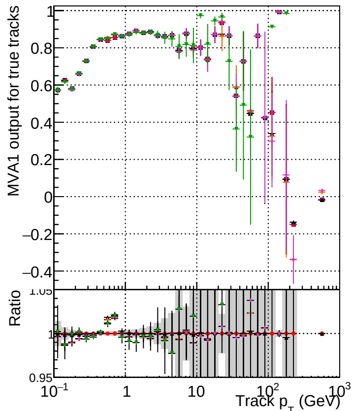
DOM original originalvector_1000evt DOM original_1000evt DOM fitted4_1000evt DOM fit cpeok_1000evt DOM fit cpeok SORTRZ2_1000evt DOM fit cpeok SORTRZ2 TESTOUTLIER2_1000evt
