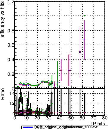
DQM original originalvector_1000evt DQM original_1000evt DQM fitted4_1000evt DQM fit_cpeOK_1000evt DQM fit_cpeOK_SORTRZ2_1000evt DQM fit_cpeOK_SORTRZ2_TESTOUTLIER2_1000evt
