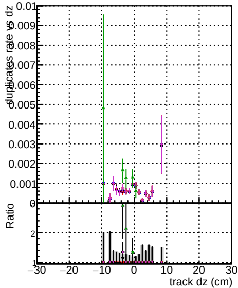
OUTLIER2 1000evt
